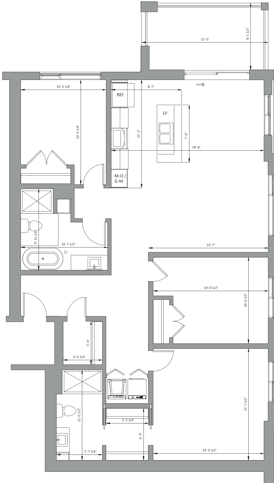
Étages 2-3
